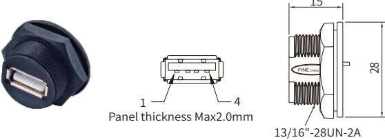
USB2.0
